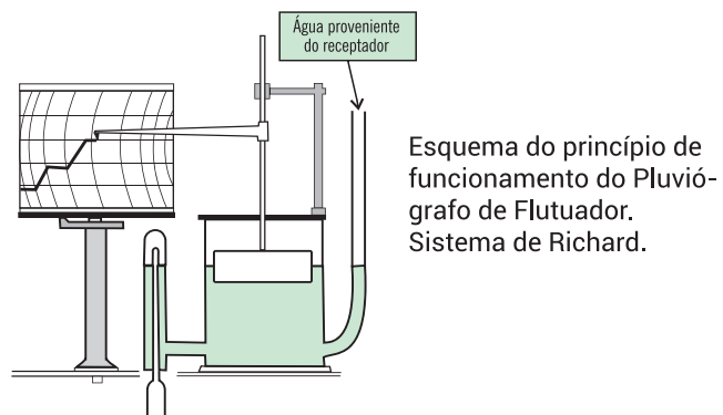
Figura 5 - Pluviógrafo
