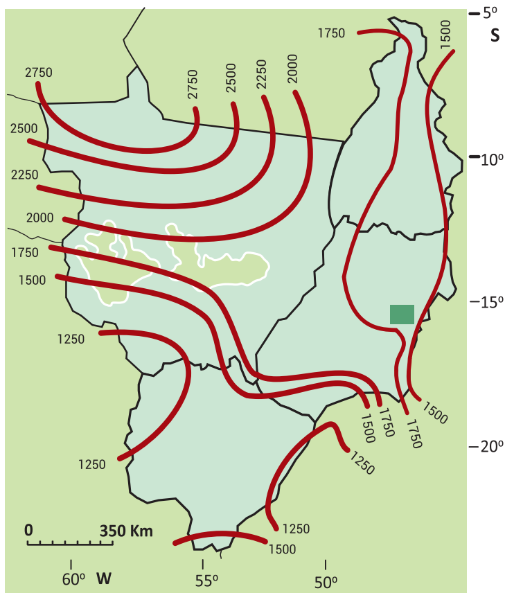
Figura 2 - Isoietas
